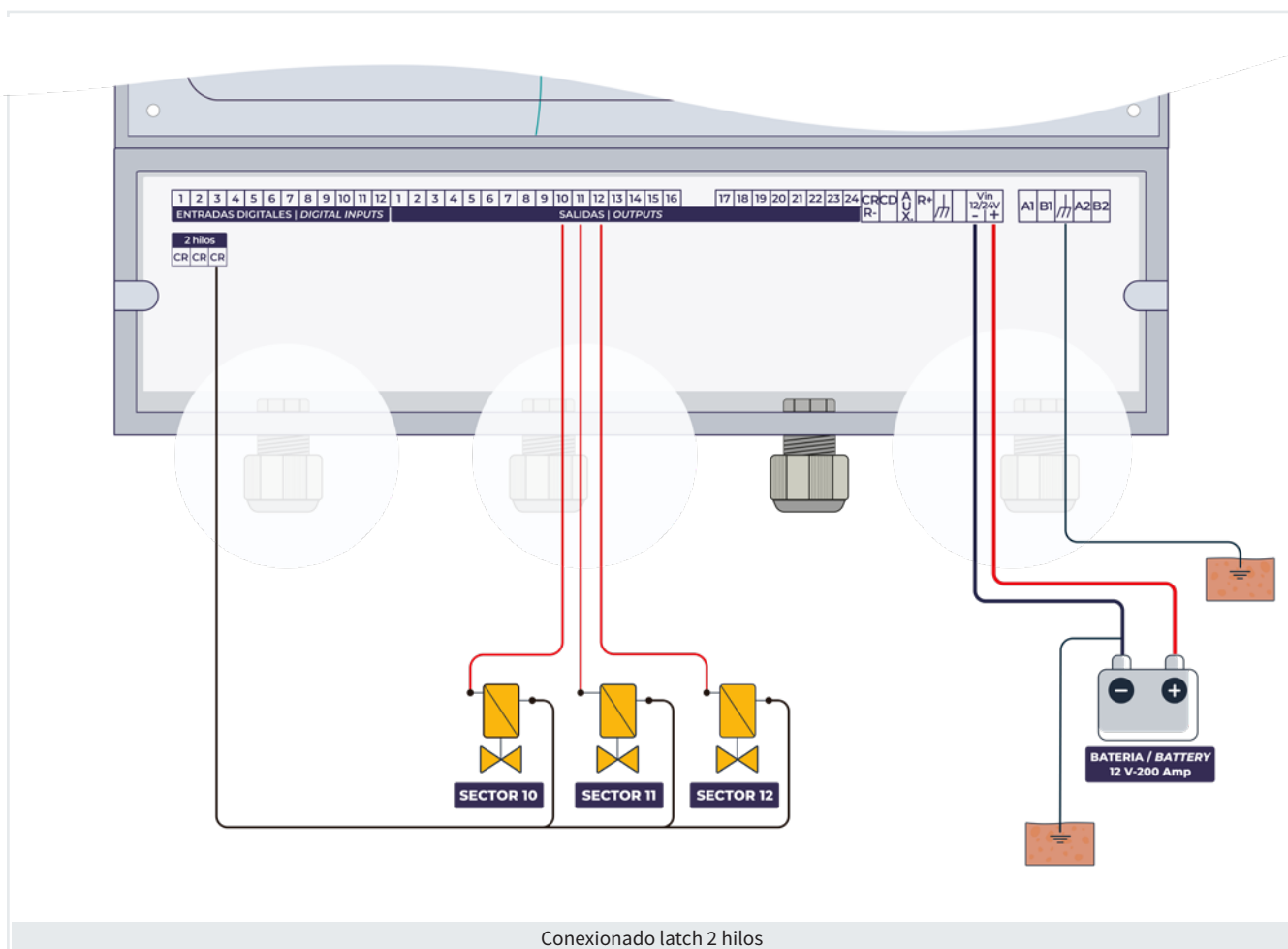
Conexionado latch 2 hilos
